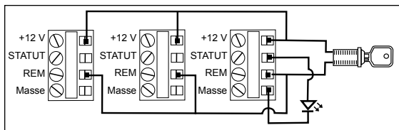
Fig. B Trois unités de PS-8RE III configurées pour le mode parallèle en continu avec voyant DEL.
