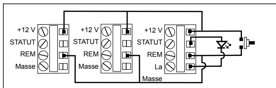
Fig. C Trois unités PS-8RE III configurées pour le mode parallèle instantané avec indicateur DEL.
